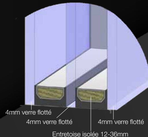
Flotteur 4mm + Flotteur 4mm + Flotteur 4mm
