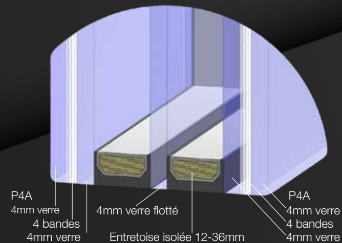
P4A + Flotteur 4mm + P4A
